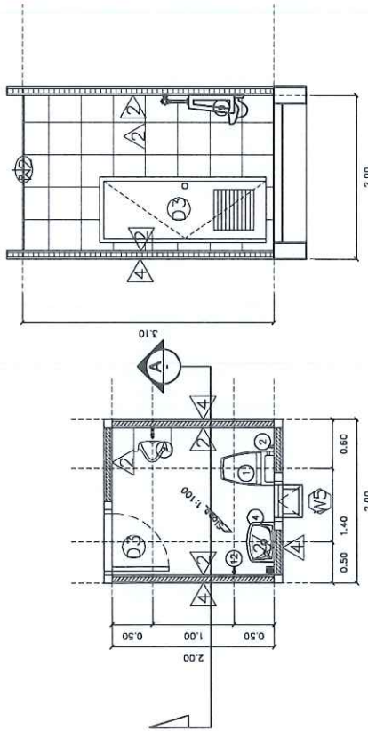
ห้องนั่งเล่นใต้ 4 F2+0.60 C2 - แปลนพื้น SCALE 1:50
