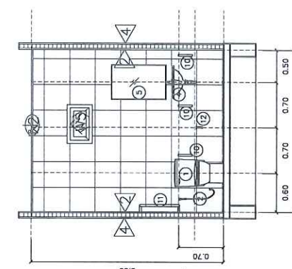
ห้องนั่งเล่นใต้ 3 F2+0.50 C2 - แปลนพื้น SCALE 1:50
